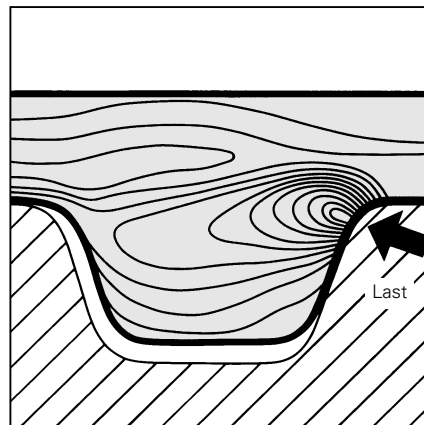
Spannungsverteilung im Trapez Zahn
