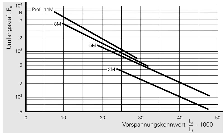
Vorspannungskennlinien
